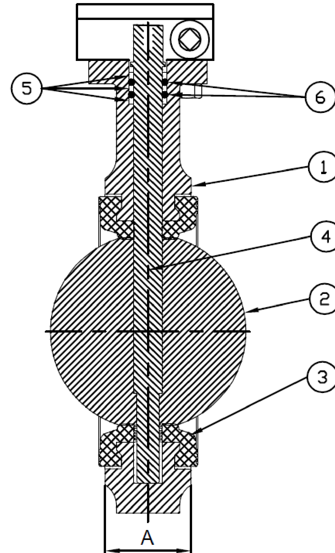
SECTION A-A
