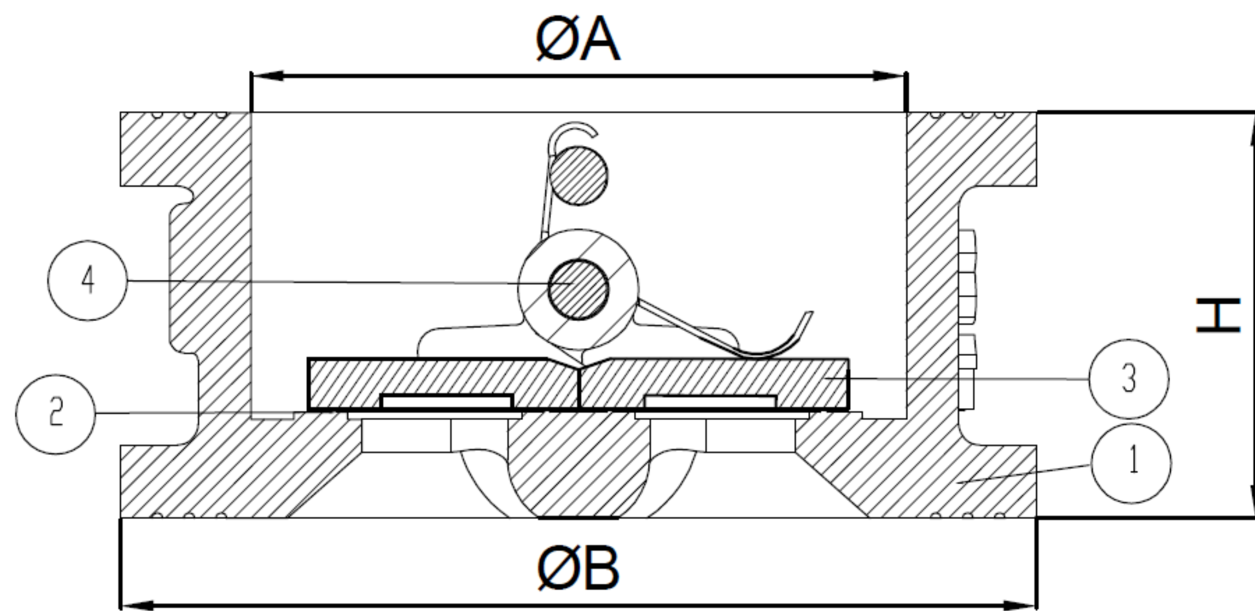
SECTION A-A
